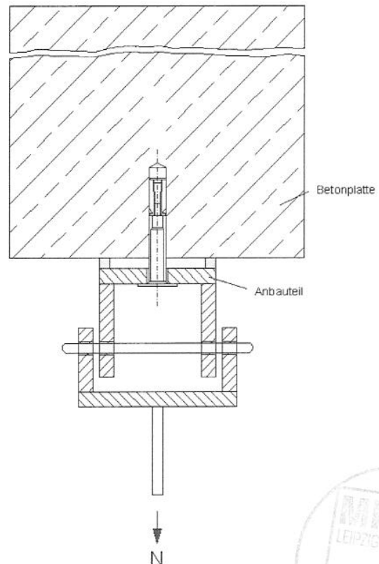
Ansicht Zugvorrichtung
