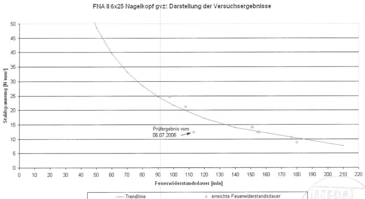
Bild 1: FNA II 6x25 Nagelkopf gvz - Darstellung der Versuchsergebnisse
