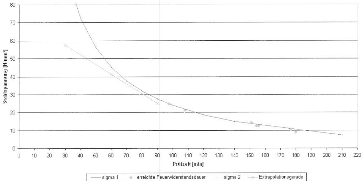
FNA II 6 x 25 Nagelkopf (gvz): Auswertung der Versuchsergebnisse
