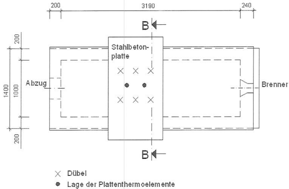
Prüföfen - Draufsicht
