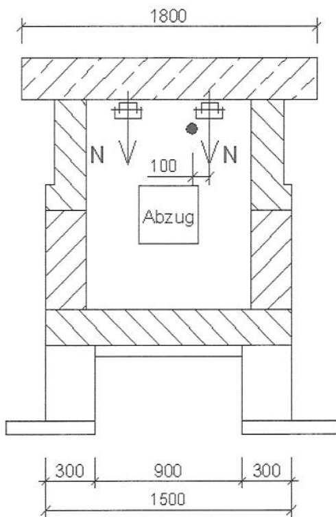
Schnitt B-B
