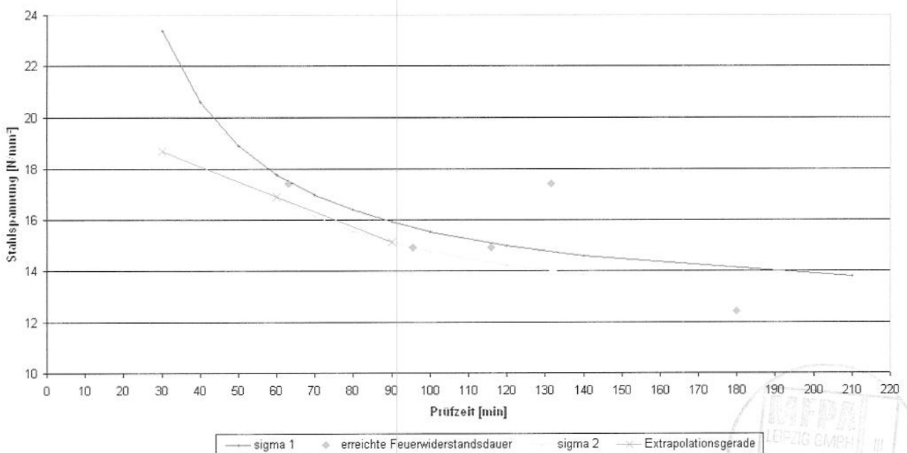
FNA II 6 x 25 Gewindebolzen M6 (gvz): Auswertung der Versuchsergebnisse
