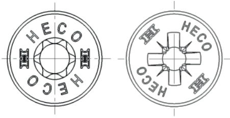
Kopfkennzeichnung bei d = 3,5 bis 6,5 mm aller Kopfausführungen. Kopfformen auch ohne Beschriftung möglich.
