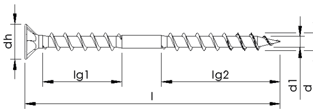
Unterkopfgewinde ohne Variation, ohne Schaftrippen, mit Spitzenverzahnung
