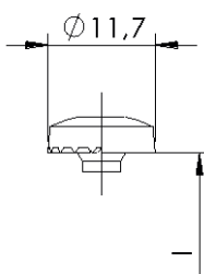
Panhead mit und ohne Unter- kopffräsrippen
