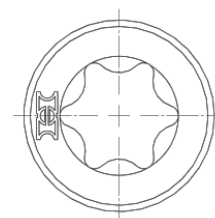
Kopfkennzeichnung bei d = 4,5 bis 10,0 der Ausführungen: Zylinderkopf, Zylindersenkkopf. Genannte Kopfform auch ohne Beschriftung möglich.
