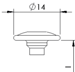
Lintentellerkopf mit aufgedicktem Schaft
