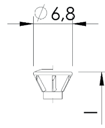
Flachsensenkopf 60 / 75° mit und ohne Linse, mit und ohne Fräsrippen
