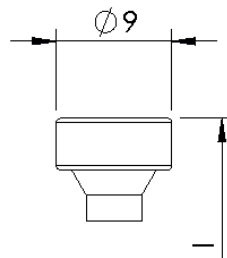
Zylindersenkopf
