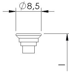
Stufenkopf
