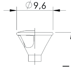
Flachsenkopf 60 / 75° mit und ohne Linse, mit und ohne Frästaschen
