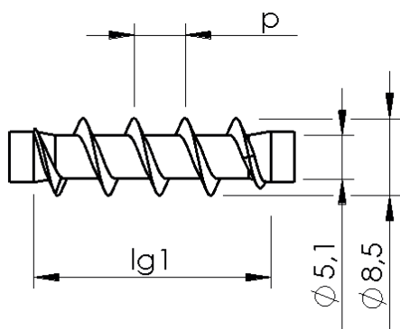
Unterkopfgewinde
