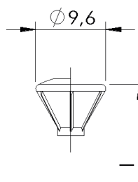
Flachsenkopf 60° / 75° mit und ohne Linse, mit und ohne Fräsrippen
