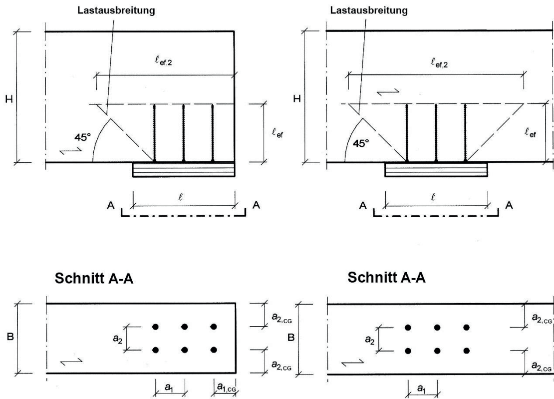
Abbildung 4: Verstärktes Endauflager (links) und verstärktes Zwischenaflager (rechts)
