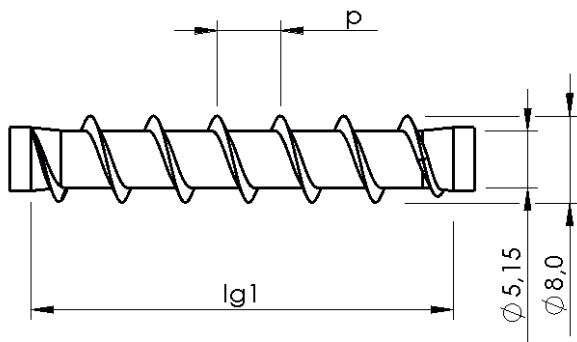
Unterkopfgewinde
