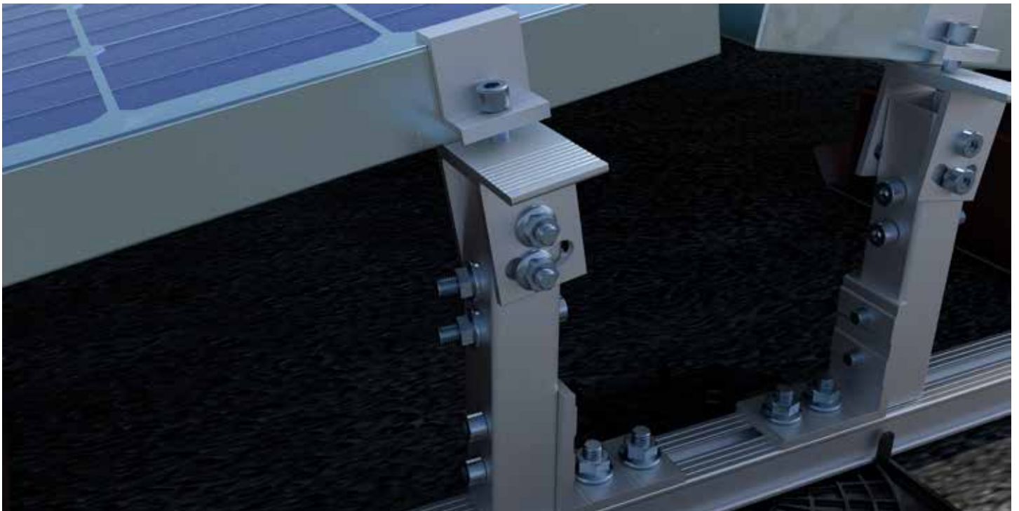
Gelenk für Modulaufständerung hinten im montierten Zustand
